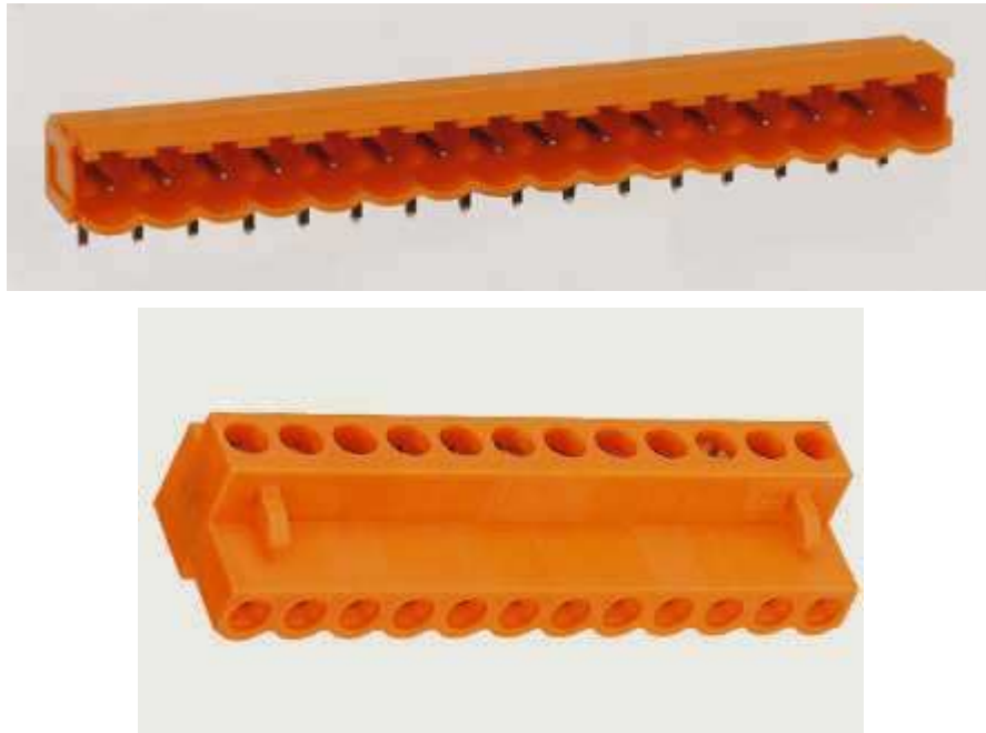
Figure 8.2. Connecteurs débrochable Weidmüller (Weid-m.jpg & Weid-f.jpg).
