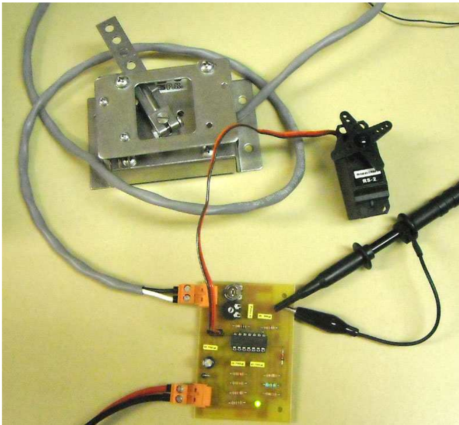
Figure 8.1. Vue de carte électronique (images-maquettes\SERVO1-22.jpg).
