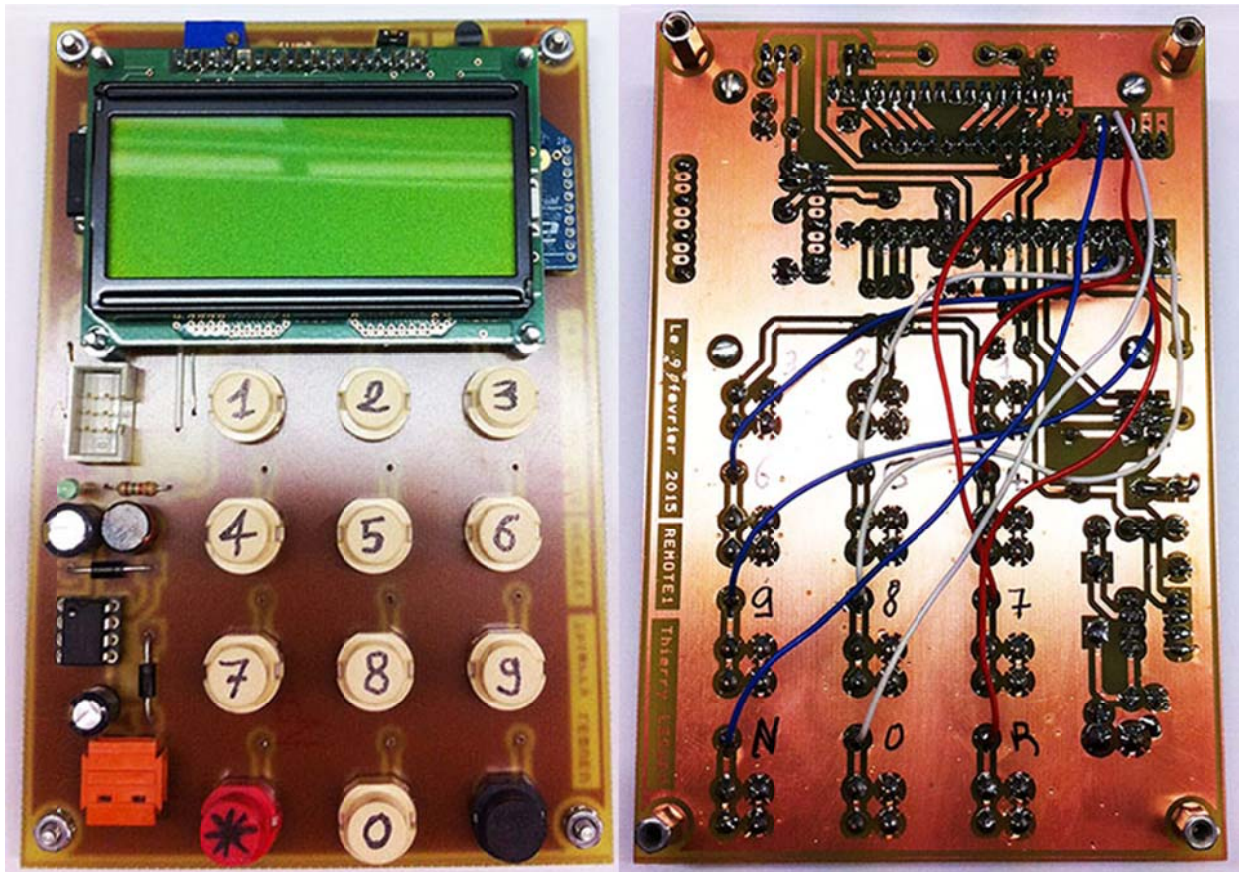
Figure 4.1. Vue de carte électronique (images-maquettes\REMOTE1-13 & 33.jpg).
