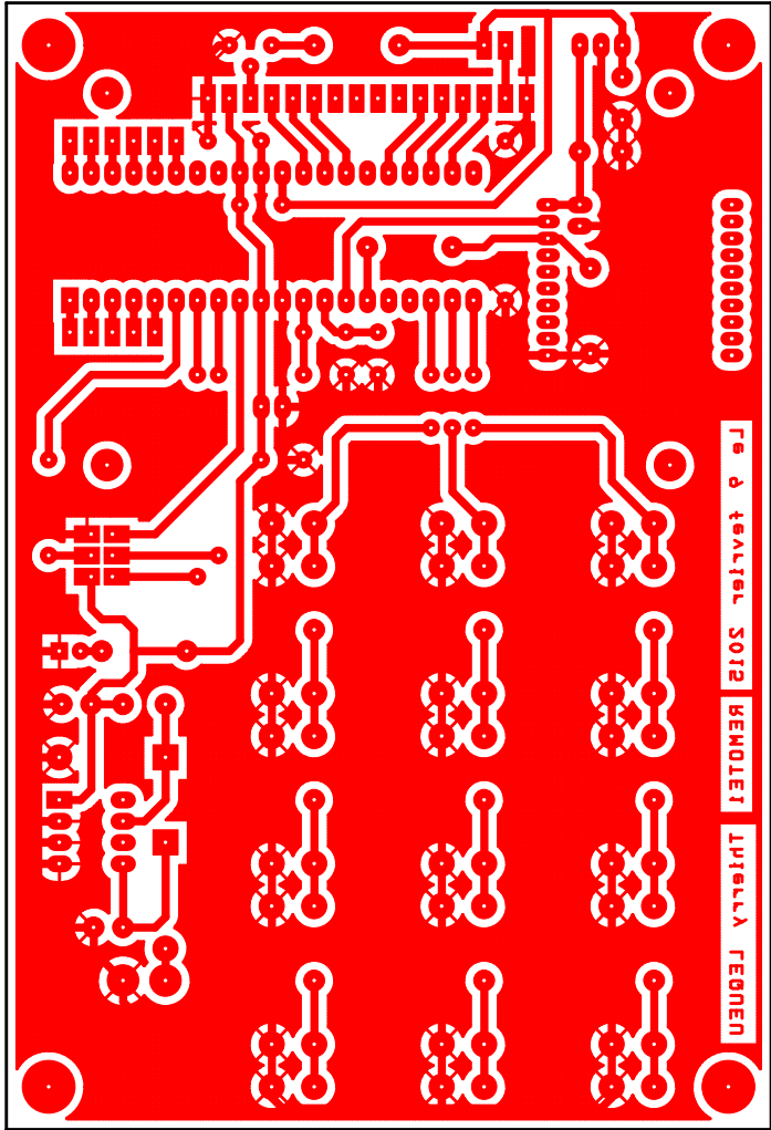
Face BOT
