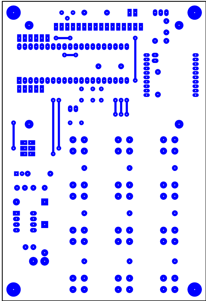
Face TOP
