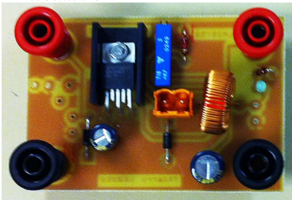
Figure 3.16. Vue de carte électronique version ajustable (images-maquettes\lm2575e-43.jpg).
