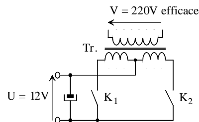
Figure 3.6. Principe de l'onduleur à point milieu (dessins\ond_pm.drw).
