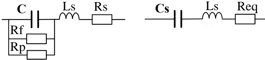
Figure 1.3. Schémas équivalents d'un condensateur (dessins\capa1.drw).
