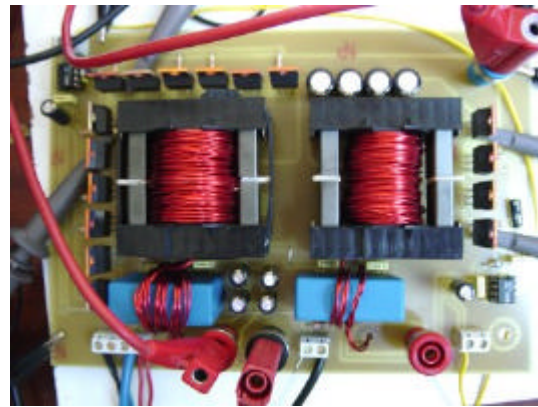
Figure 3.7. Convertisseur 12V vers 51V / 250 W (images-maquettes\12VDC51V-12.jpg).
