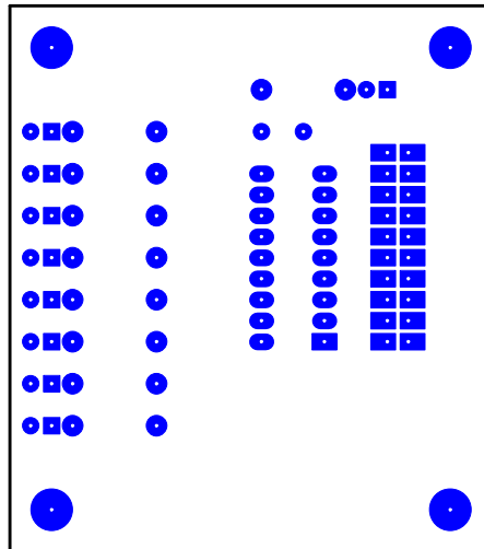
Face TOP
