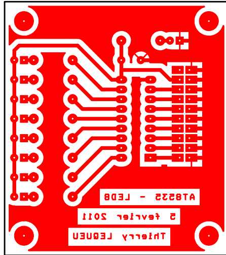
Face BOT
